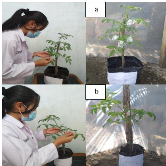
Lampiran 6. Uji Postulat koch pada daun tanaman tomat; (a) DTT I dan (b) DTT II.
